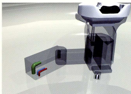
配管カバー内で立ち上げた場合
