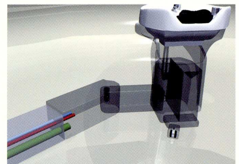
床上転がし配管の場合
