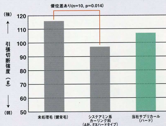
図3. ダメージ度の比較 (毛髪引張切断強度試験) 図1で評価した毛髪を使用
